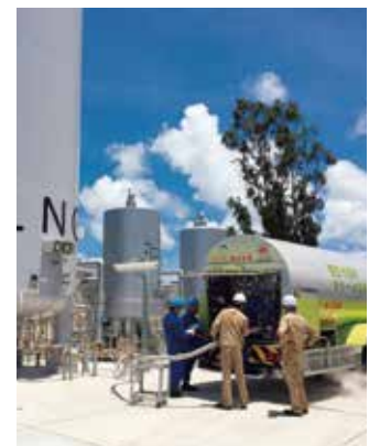
▲アワセ天然ガス供給センター
