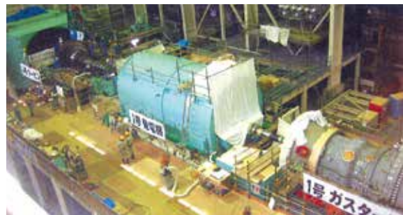
吉の浦火力発電所 蒸気タービン・発電機・ガスタービン据付
