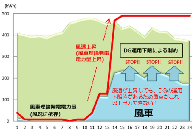
図. MGセット導入による再エネ最大化運転イメージ
