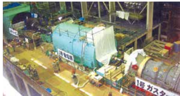
吉の浦火力発電所 タービン分解点検
