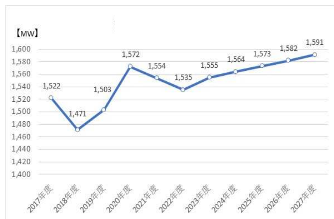
図 2-2《需要電力（送電端）》
