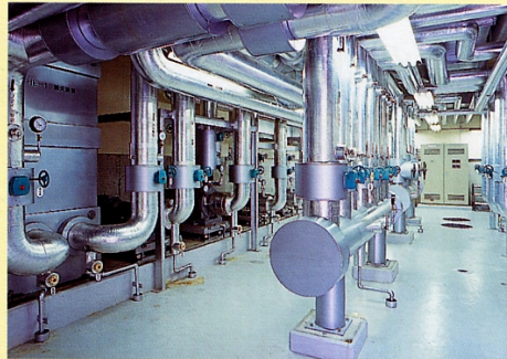
蓄熱システム(沖縄県公文書館)
