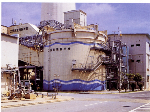
排煙脱硫装置（具志川火力発電所）
